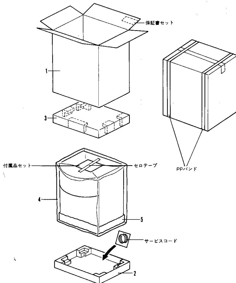
梱包図の部品表
