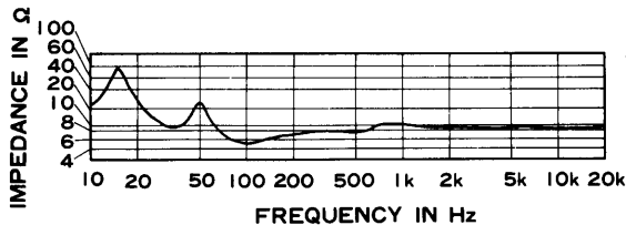
インピーダンス特性
