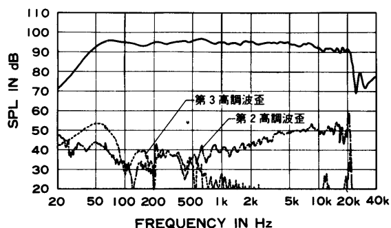
指向周波数特性
